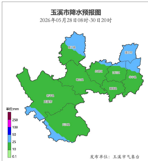
图1 玉溪市5月28日至5月30日累计降水预报图
